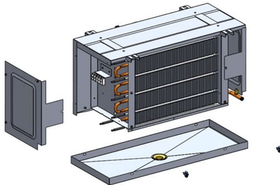
Figura 7 - Soltar a lateral e bandeja
