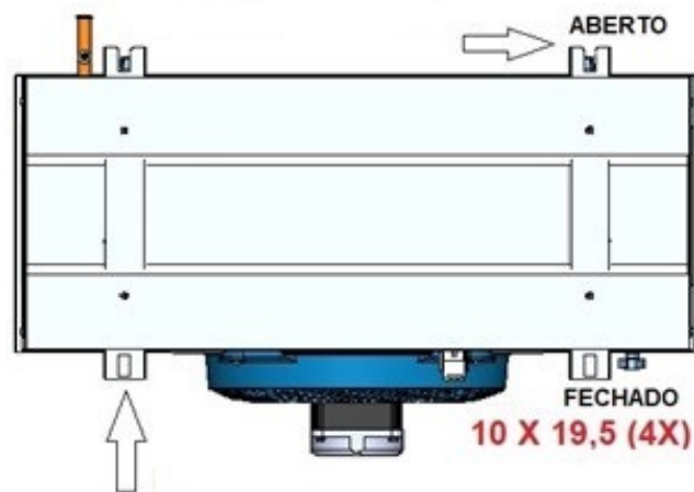
Figura 2 – Suporte de fixação
