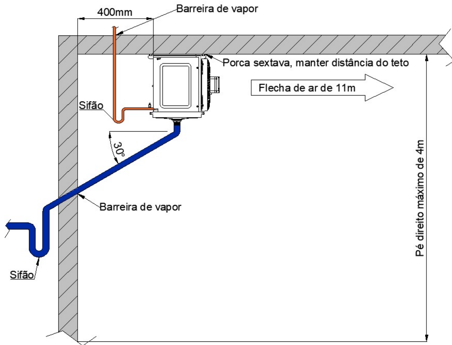
Figura 3 - Dreno da bandeja do evaporador e sifão na linha de sucção
