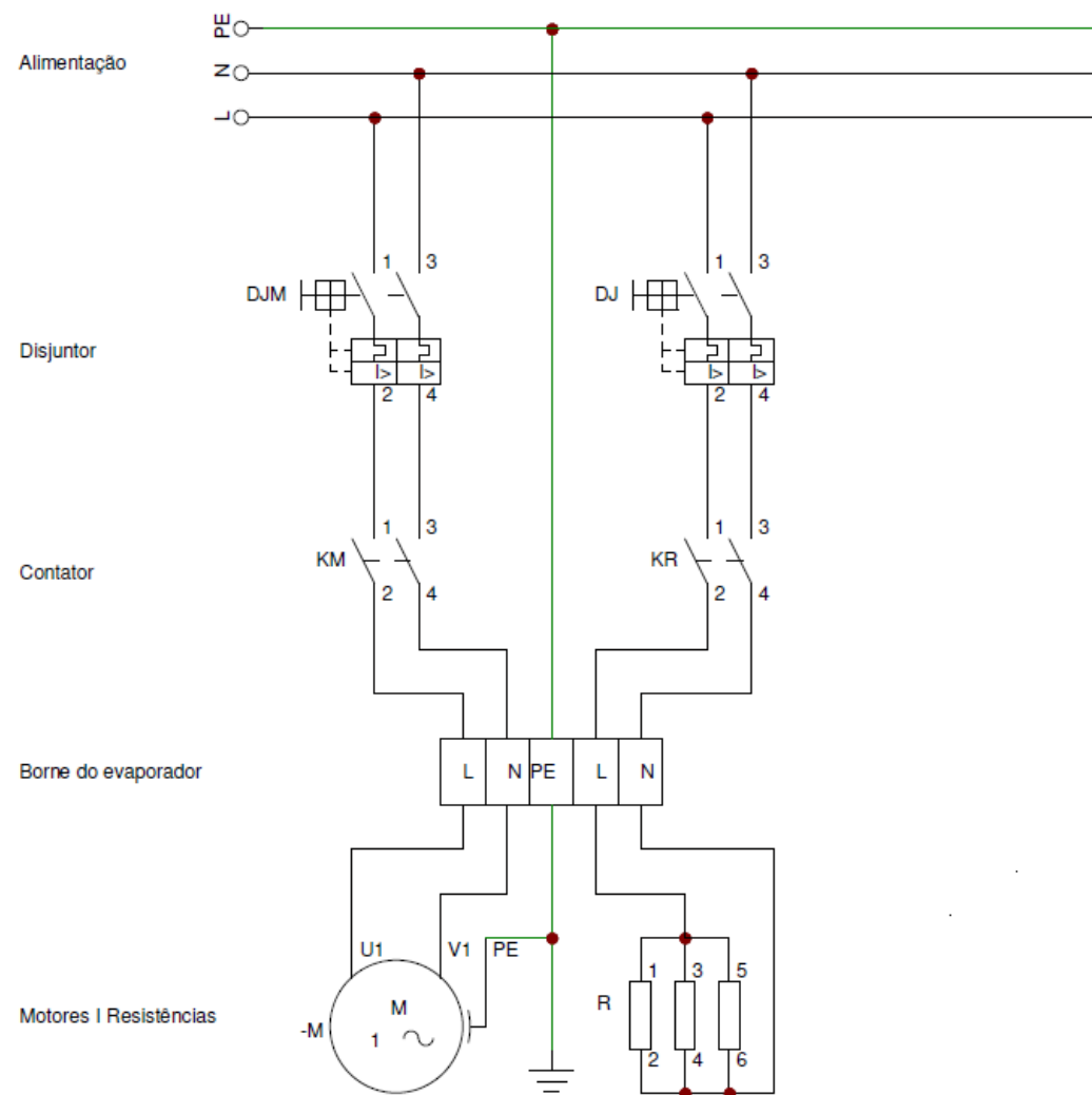
Figura 4 – Diagrama elétrico linha TRN
