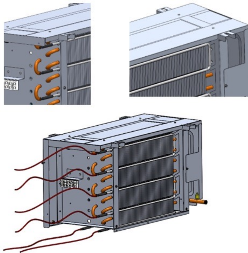
Figura 8 - Colocar as resistências de aletado nos rasgos das aletas
