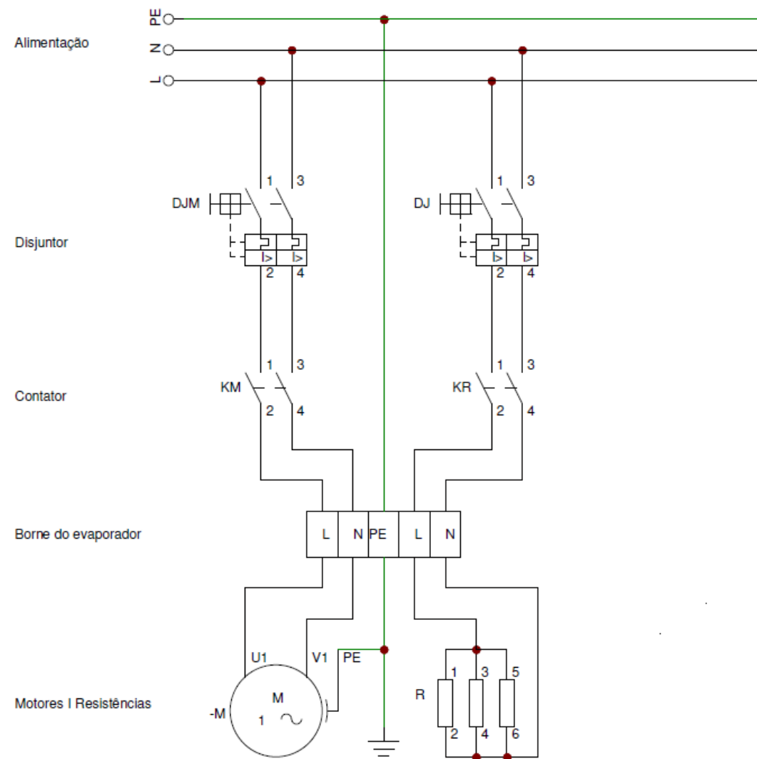
Figura 4 – Diagrama elétrico linha TRS
